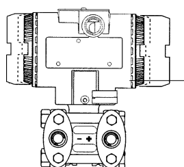
Датчик 2600Т Тх категория 1G EEx ia
