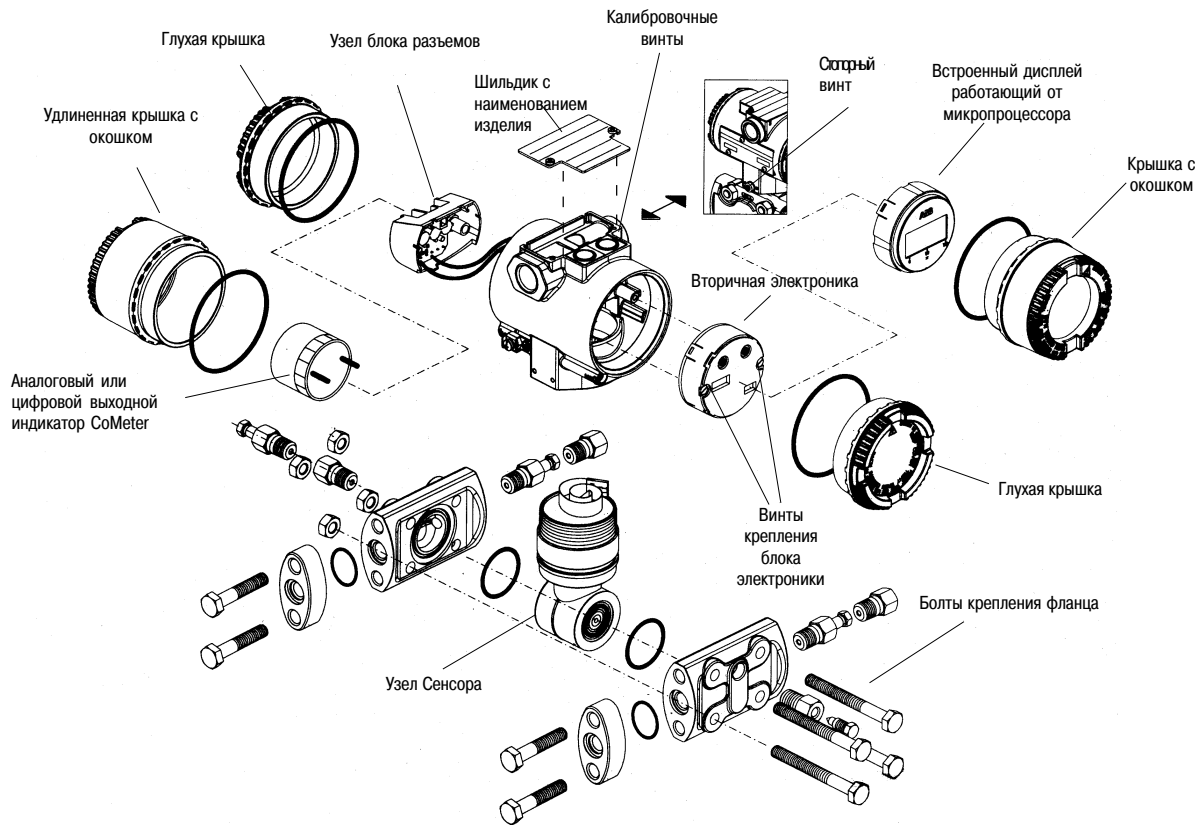
Рис. 13б - Составные части датчика для модели 264BS
