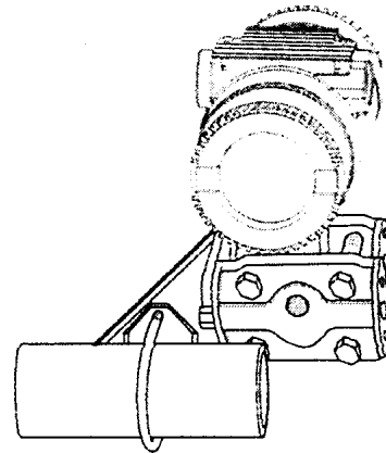
Крепление на горизонт. трубе диаметром 2 дюйма
