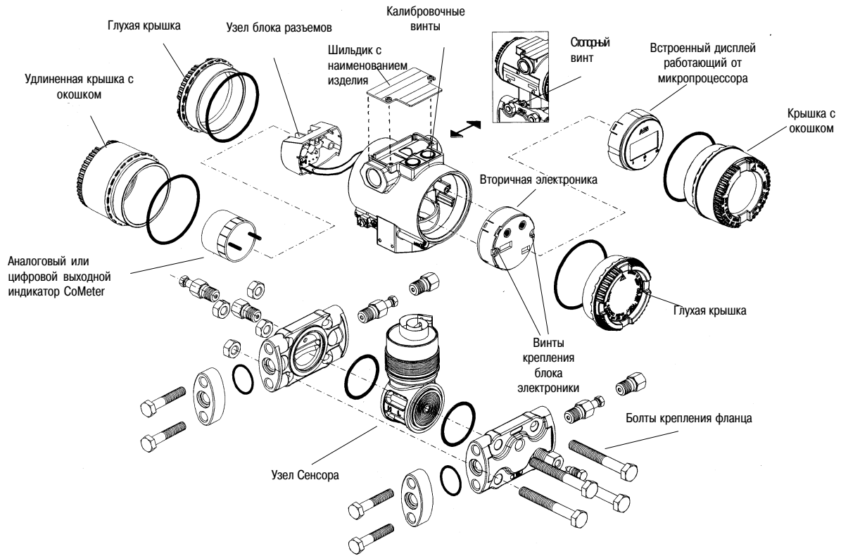
Рис. 13а - Составные части датчика для моделей 262DS/PS/VS и 264DS/PS/VS
