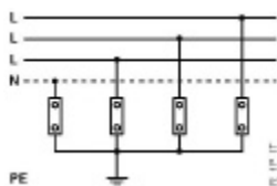
IT - TT - TNS
