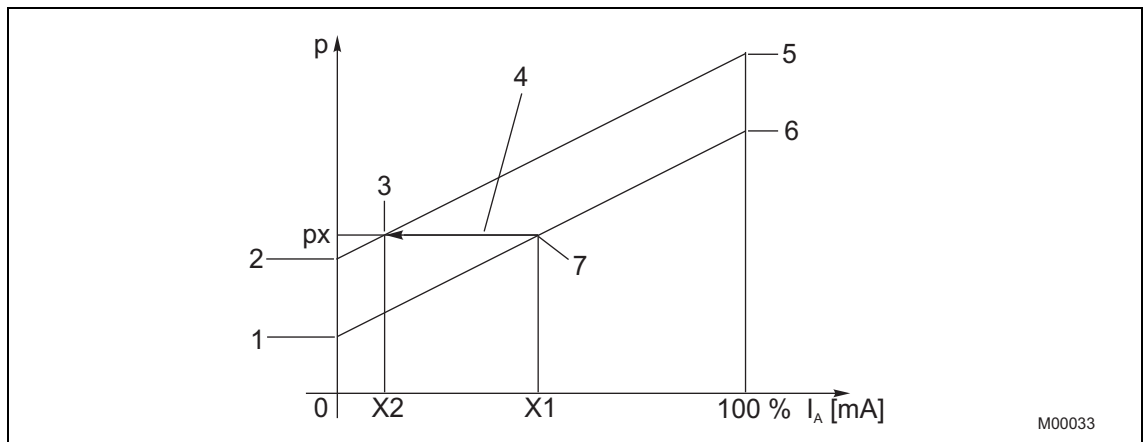
Fig. 20: Offset shift
