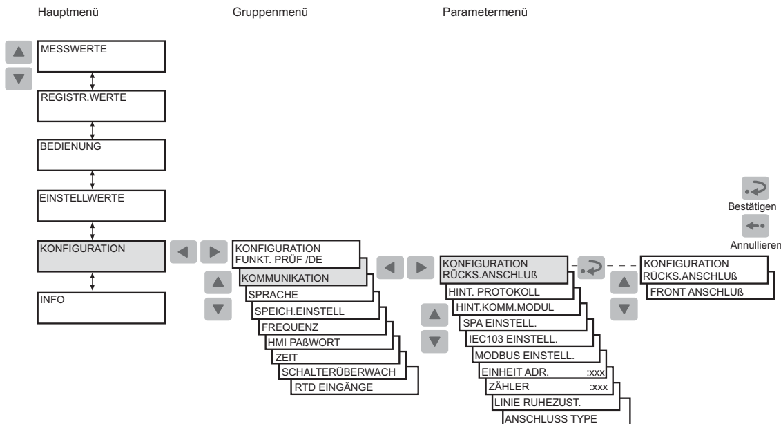
Abb. 4.1.11.-1 Umschalten zwischen frontseitigem und rückwärtigem Anschluss
