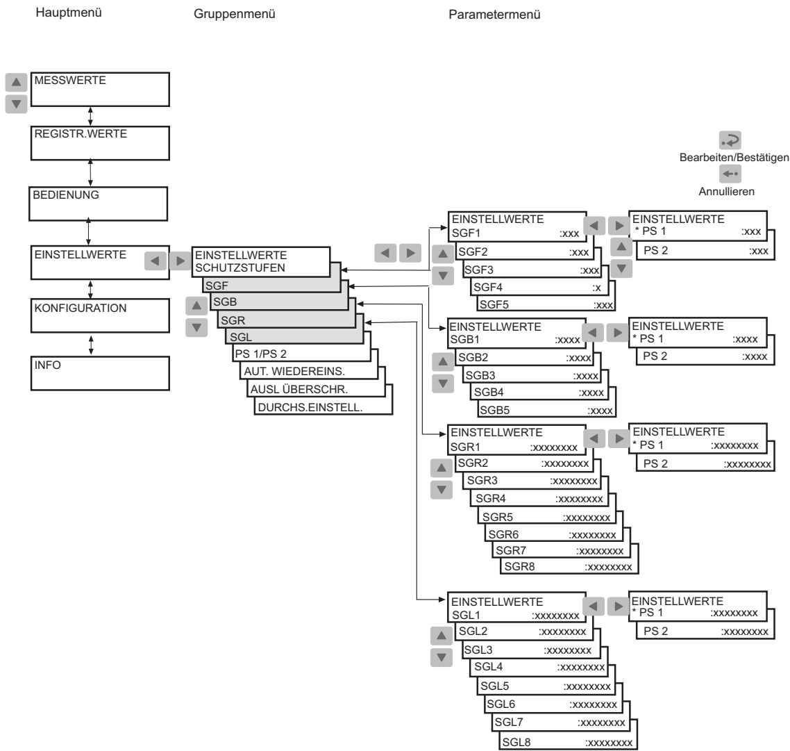
Abb. 4.2.2.2.-3 Einstellungen für Schaltergruppen
