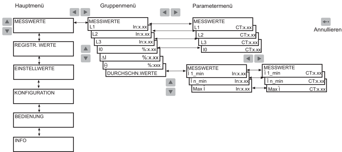
Abb. 4.2.1.2.-1 Kontrollieren der Messungen
