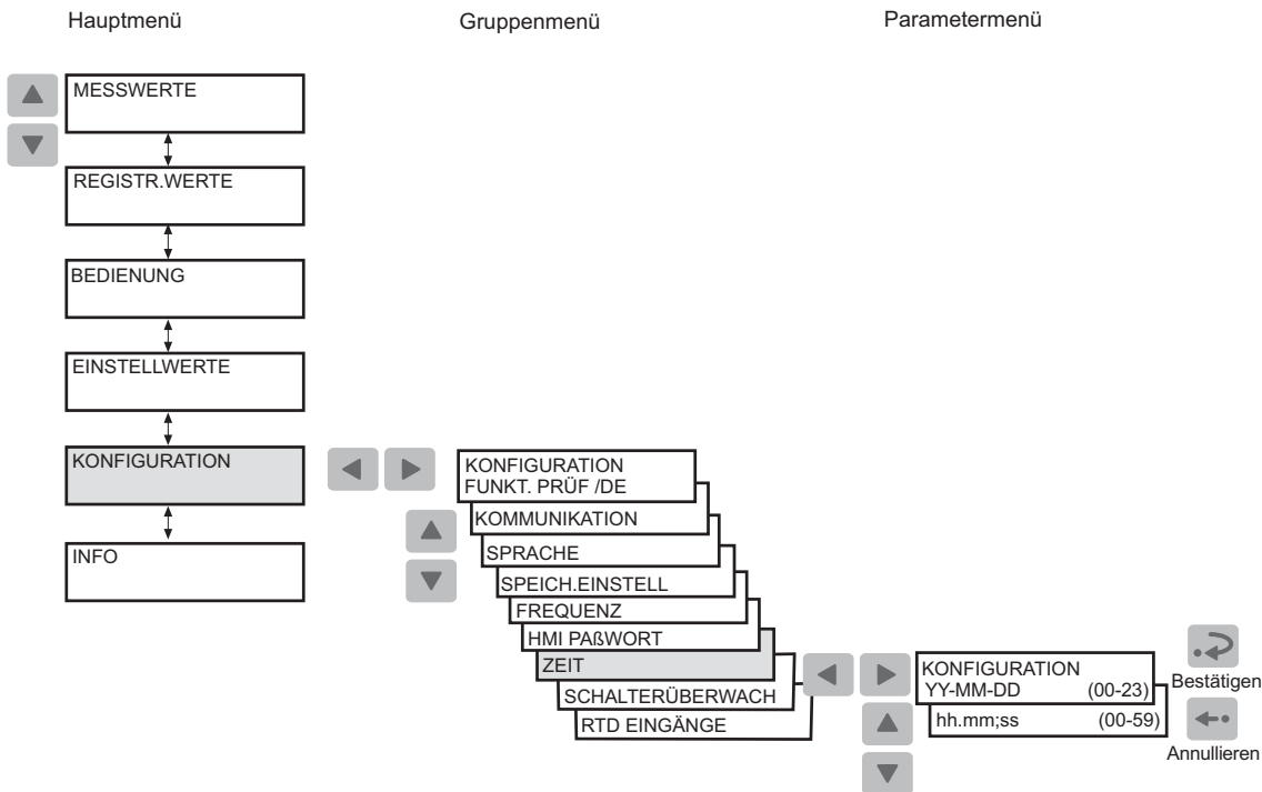
Abb. 4.1.9.-1 Einstellung der Echtzeituhr
