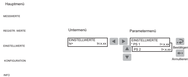
Abb. 4.2.2.2.-1 Einstellung der Parameter in den Einstellgruppen 1 und 2
