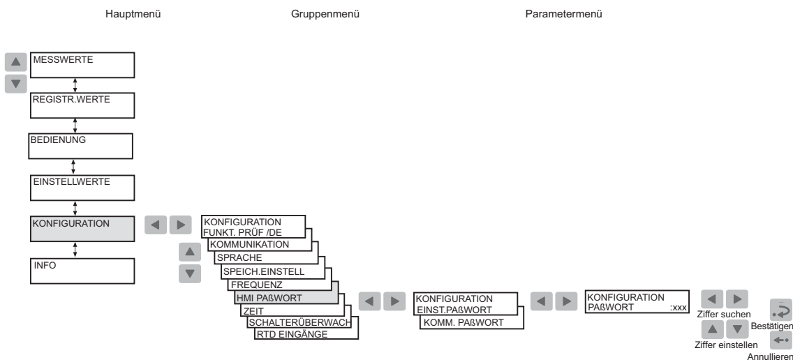
Abb. 4.1.6.-3 Änderung des MMS- Einstellungspasswortes und des MMS- Kommunikationspasswortes
