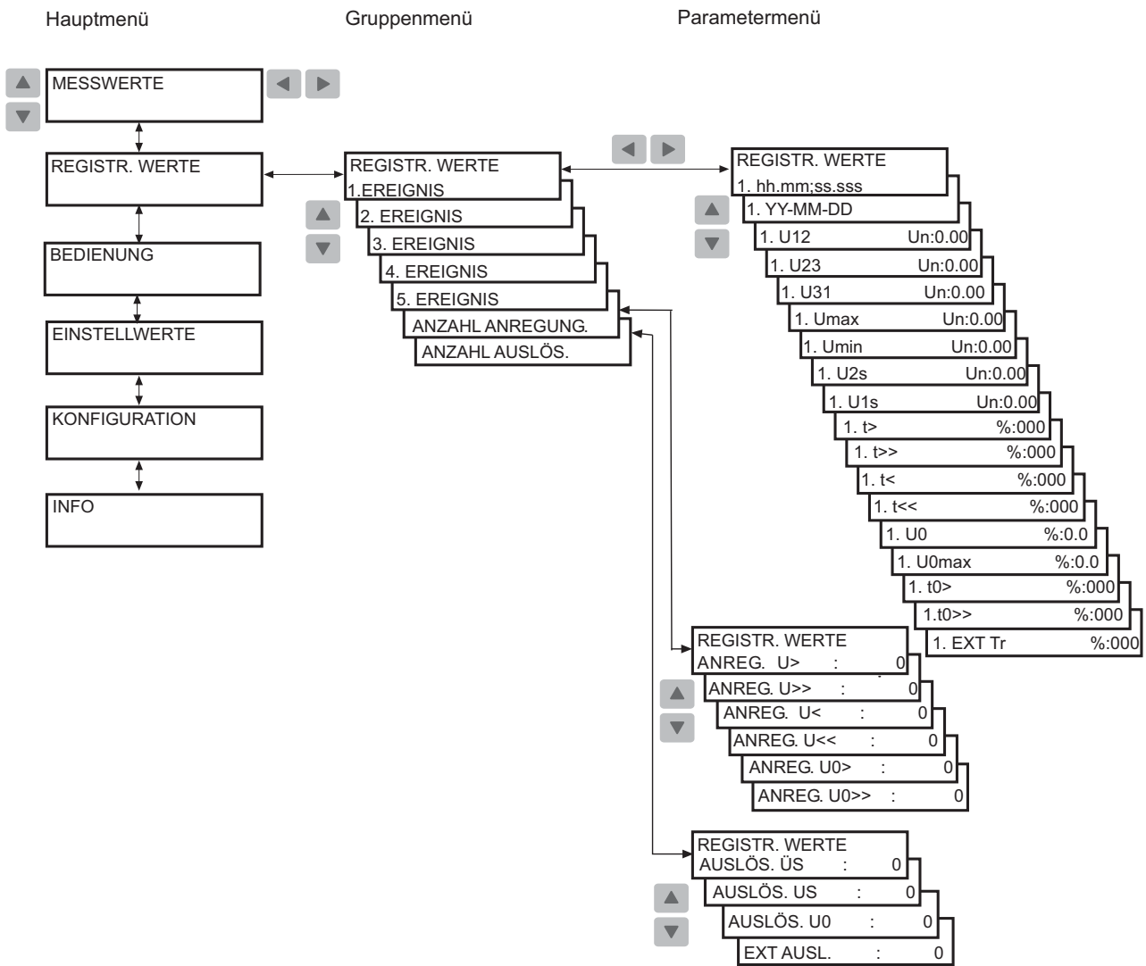
Abb. 4.2.1.3.-1 Registrierte Daten
