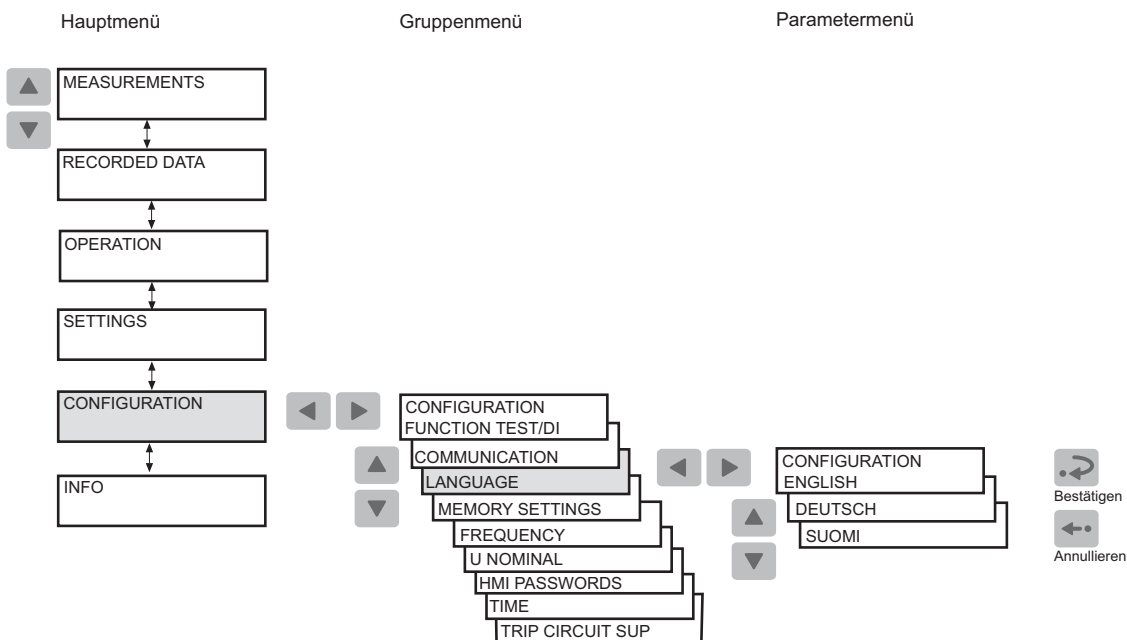
Abb. 4.2.2.3.-1 Hauptmenügruppe KONFIGURATION, Teil 1
