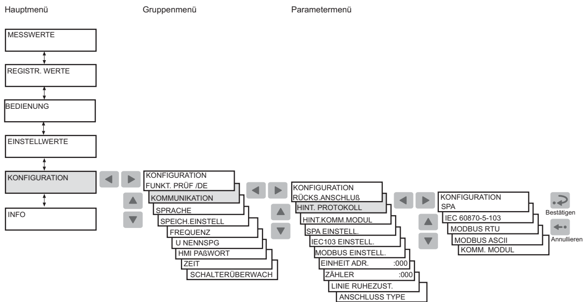
Abb. 4.1.12.-1 Wahl des Kommunikationsprotokolls für den rückwärtigem Anschluss
