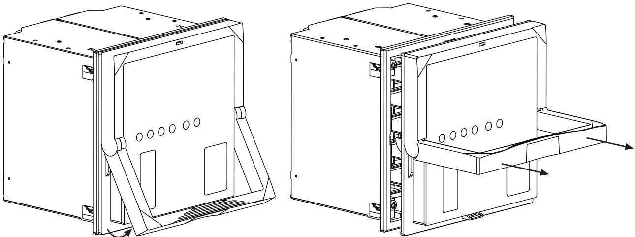
Abb. 4.4.2.-1 Entnehmen eines Einschubs aus dem Gehäuse
