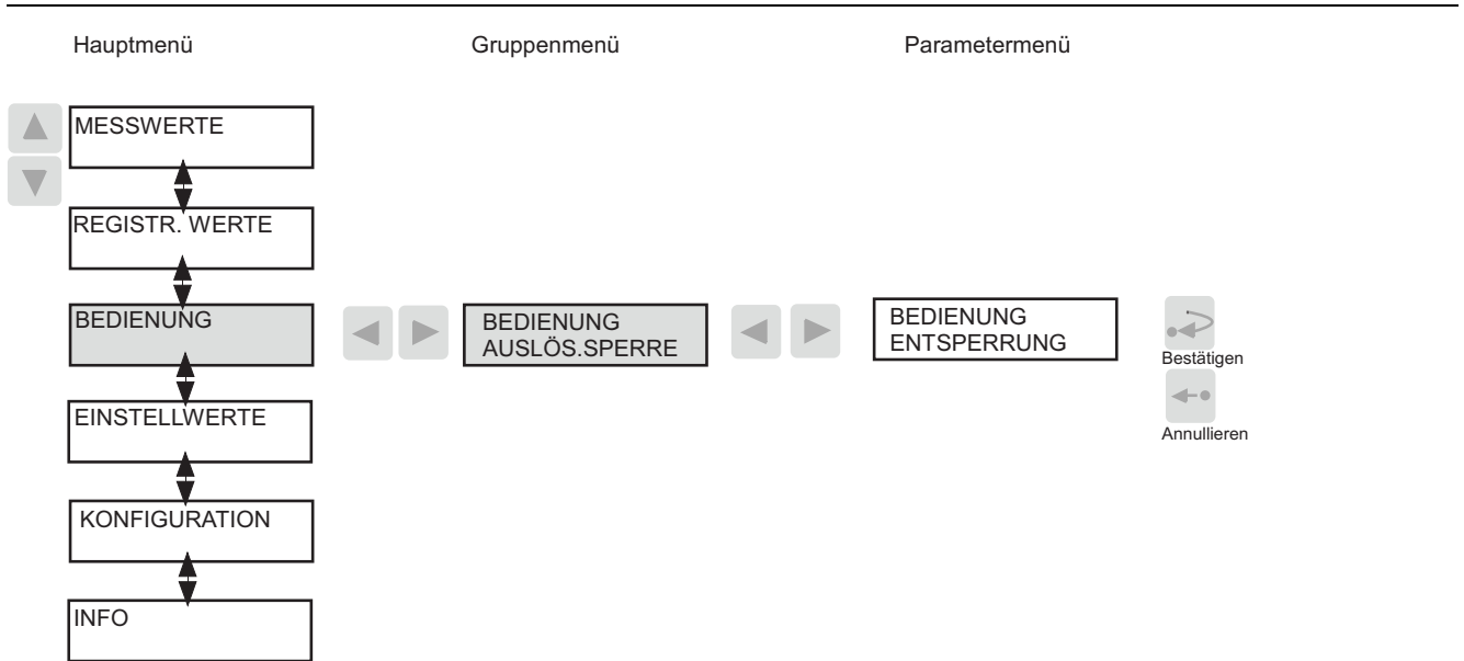
Abb. 4.1.10.-1 Bedienung
