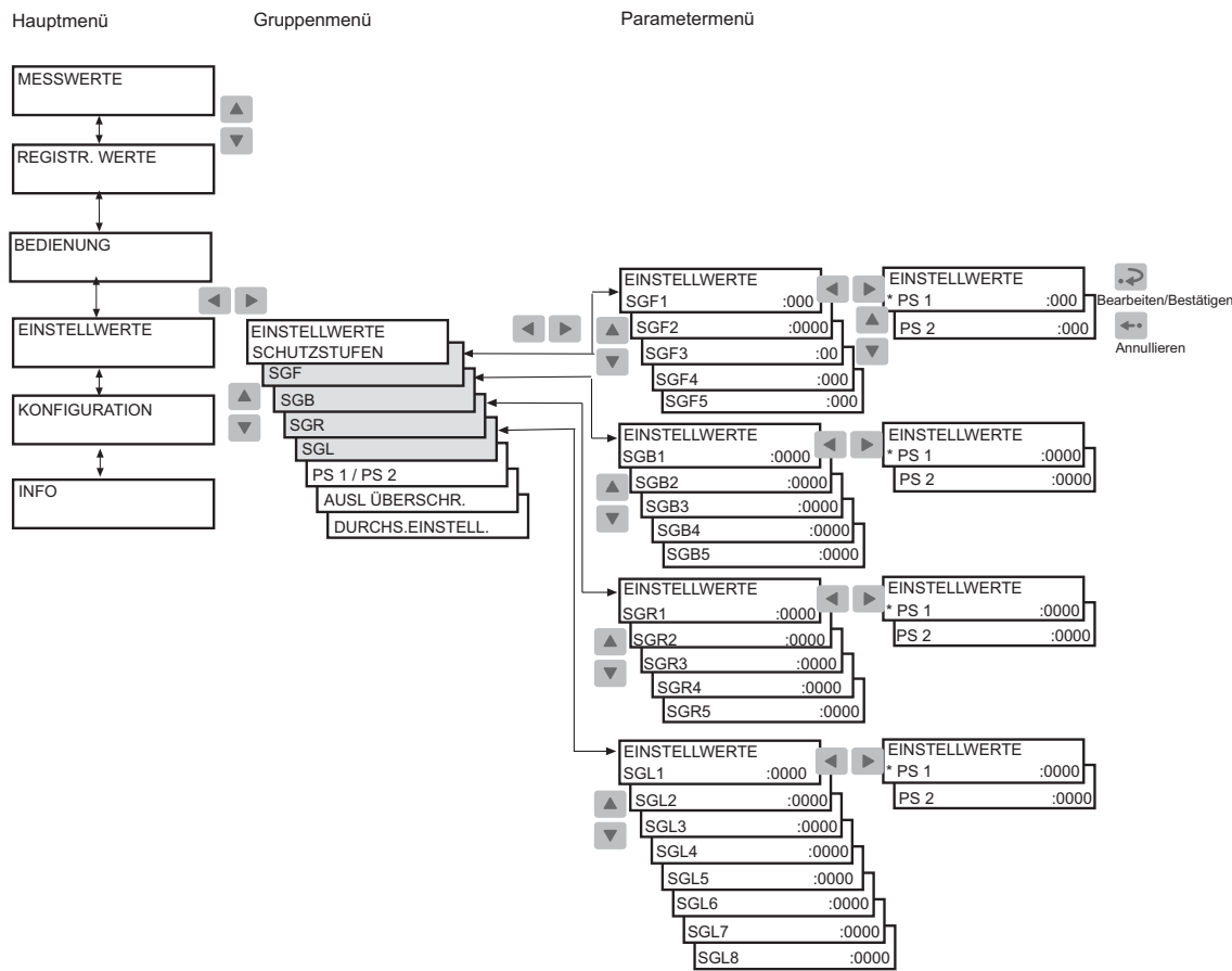
Abb. 4.2.2.2.-3 Einstellungen für Schaltergruppen
