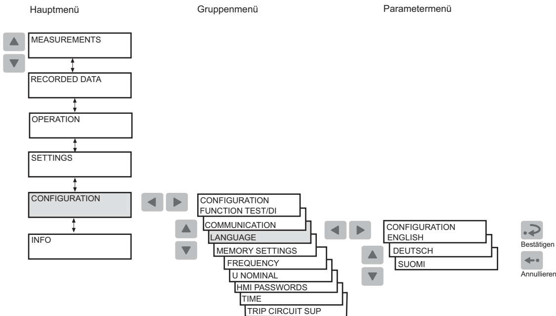
Abb. 4.1.8.-1 Wahl der Sprache
