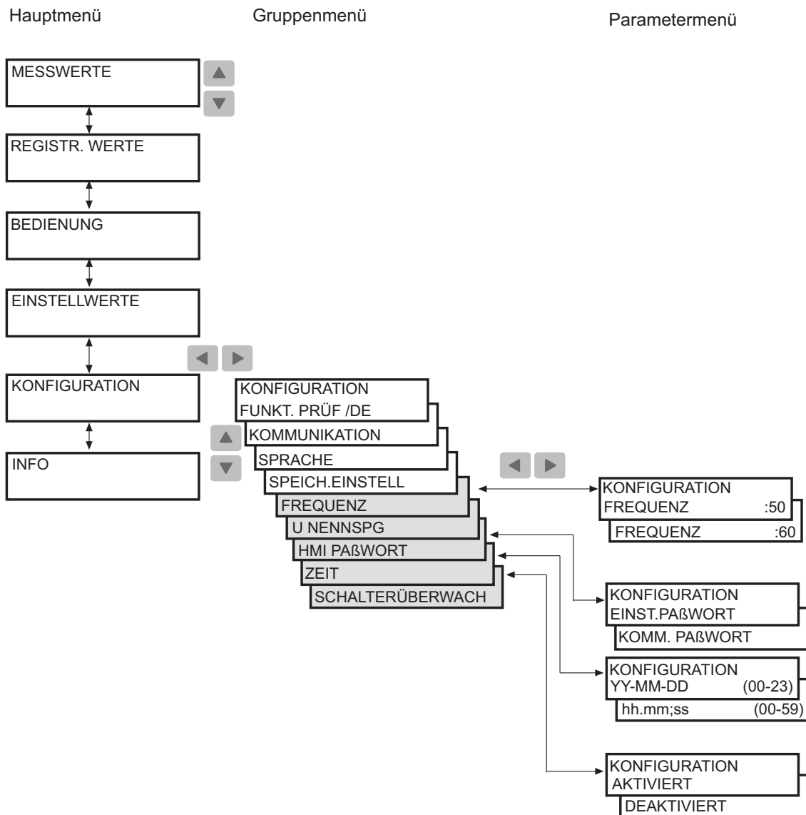
Abb. 4.2.2.3.-2 Hauptmenügruppe KONFIGURATION, Teil 2
