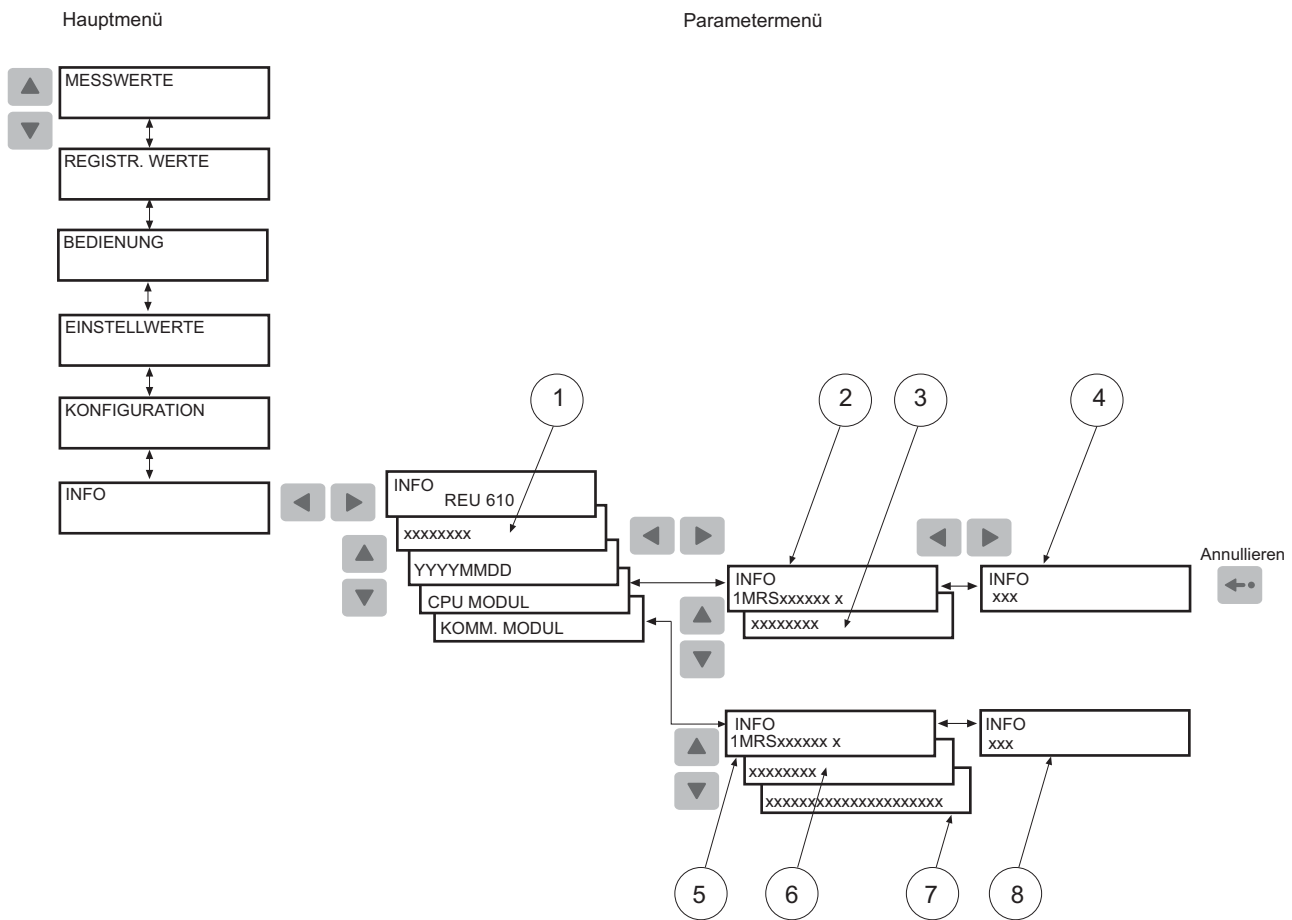
Abb. 4.2.1.4.-1 INFO
