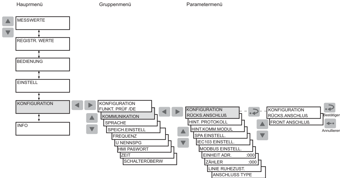
Abb. 4.1.11.-1 Umschalten zwischen frontseitigem und rückwärtigem Anschluss
