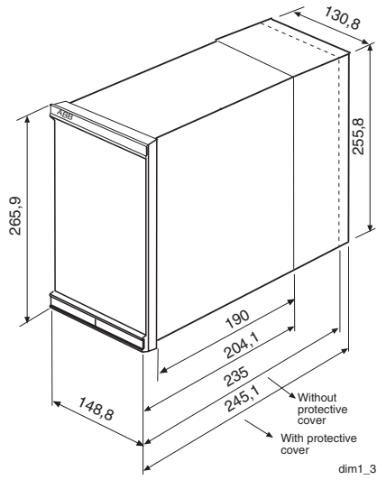
Fig. 9.-1 REA 101 dimensions
