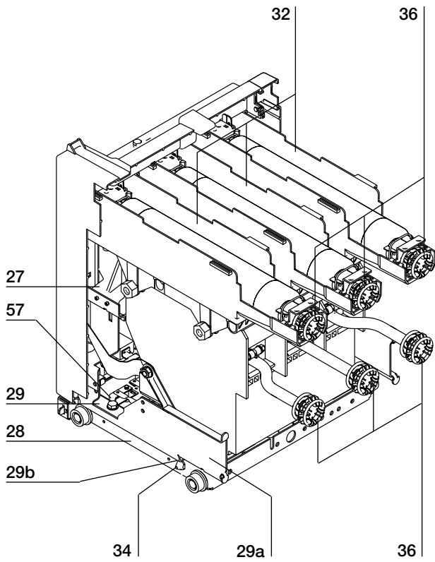
Contattore V/ZC per contenitori CBE1 e quadri ZS1
