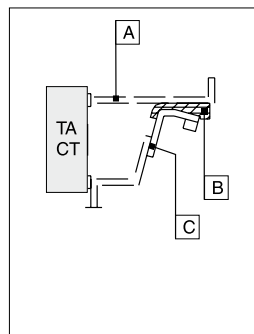
Collegamento attacco inferiore con sezionatore di terra (con TA) Lower terminal connection with earthing switch (with CT)
