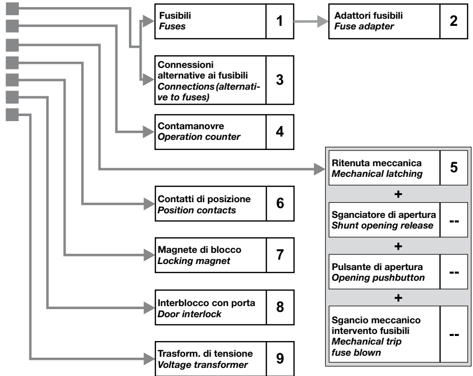
Applicazione degli accessori Application of accessories
