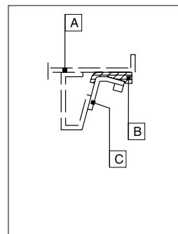
Collegamento attacco inferiore con sezionatore di terra (senza TA) Lower terminal connection with earthing switch (without CT)
