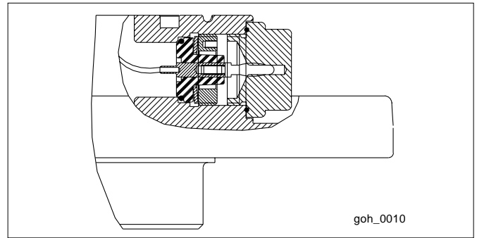
Fig. 3. Test tap
