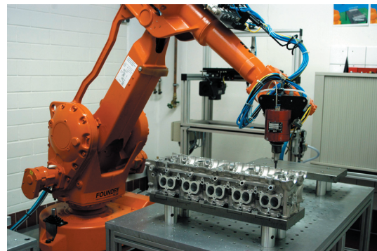
Entgraten des Zylinders zum Motorblock
