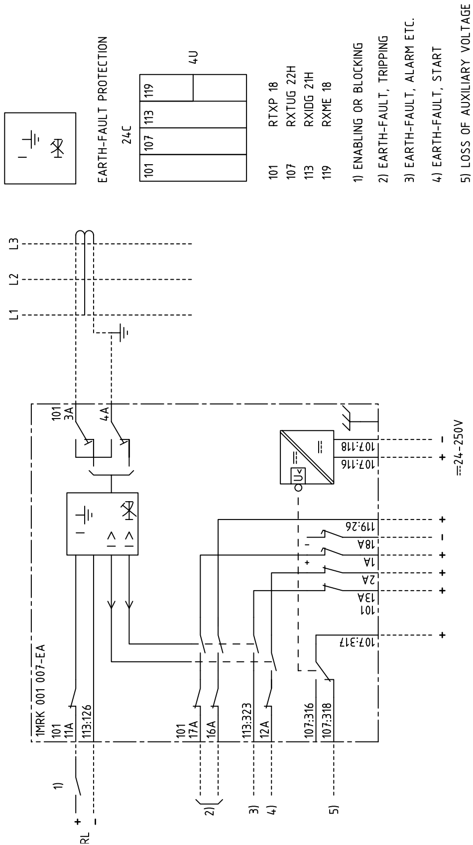
Fig. 56 Circuit diagram 1MRK 001 007-EAA
