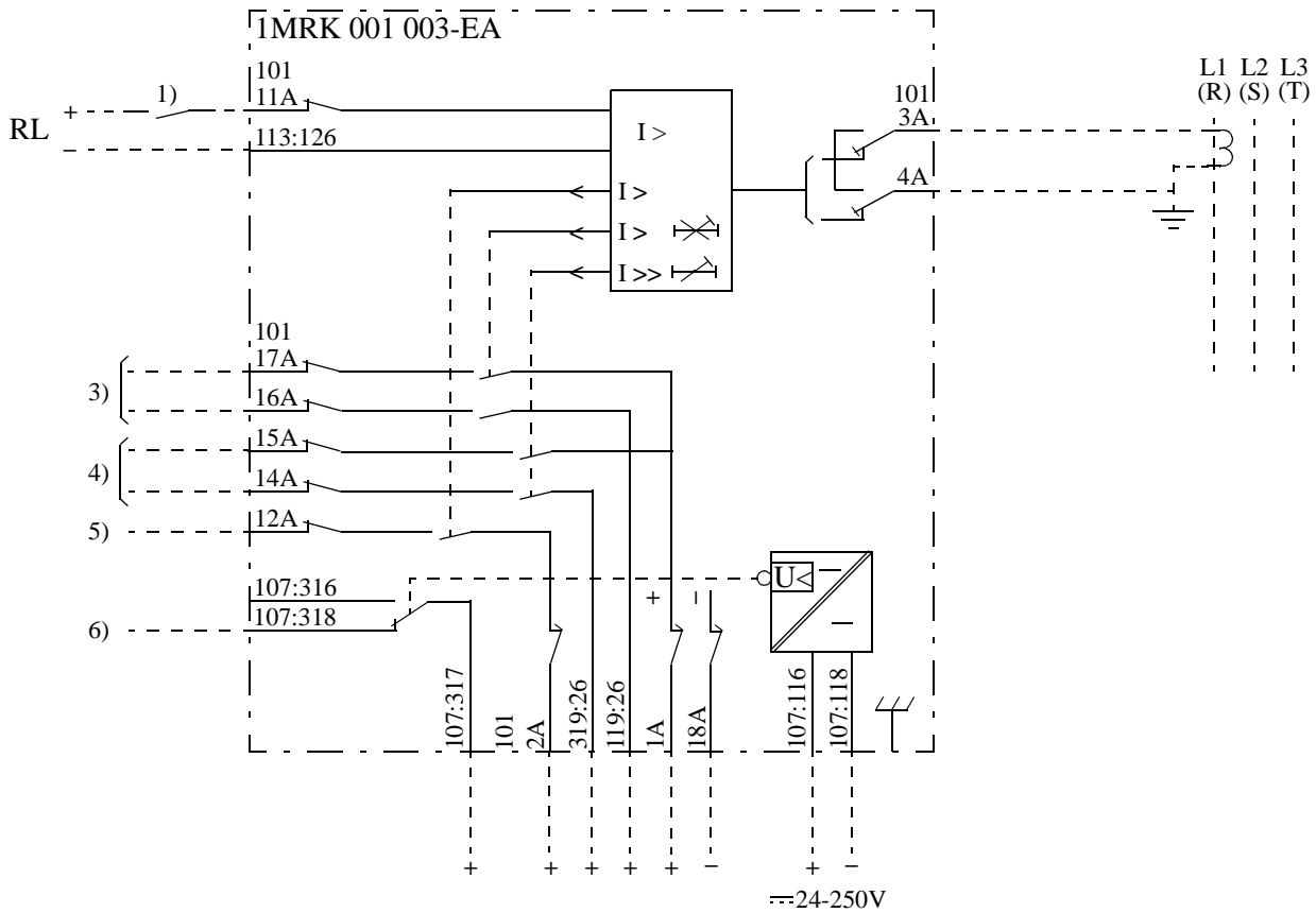
Fig. 45 Terminal diagram 1MRK 001 003-EAA
