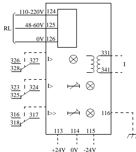
Fig. 20 Terminal diagram RXIDK 2H
